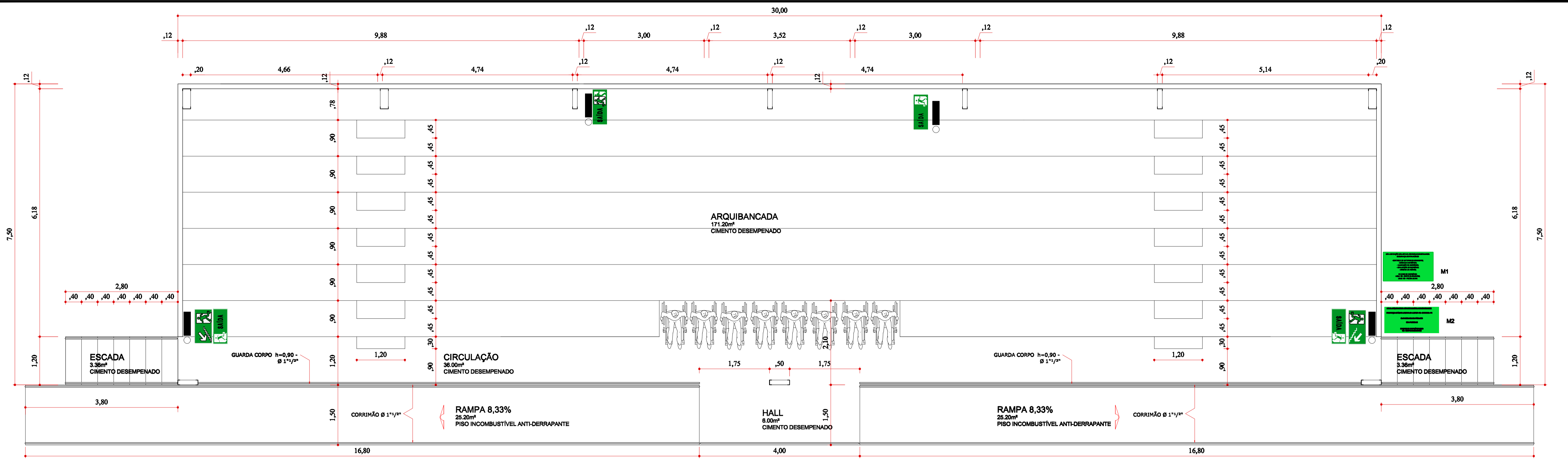
PLANTA BAIXA ESCALA 1:50 ÁREA : 288,12m²
