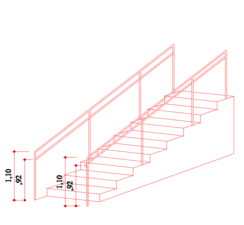
DETALHE CORRIMÕES SEM ESCALA
